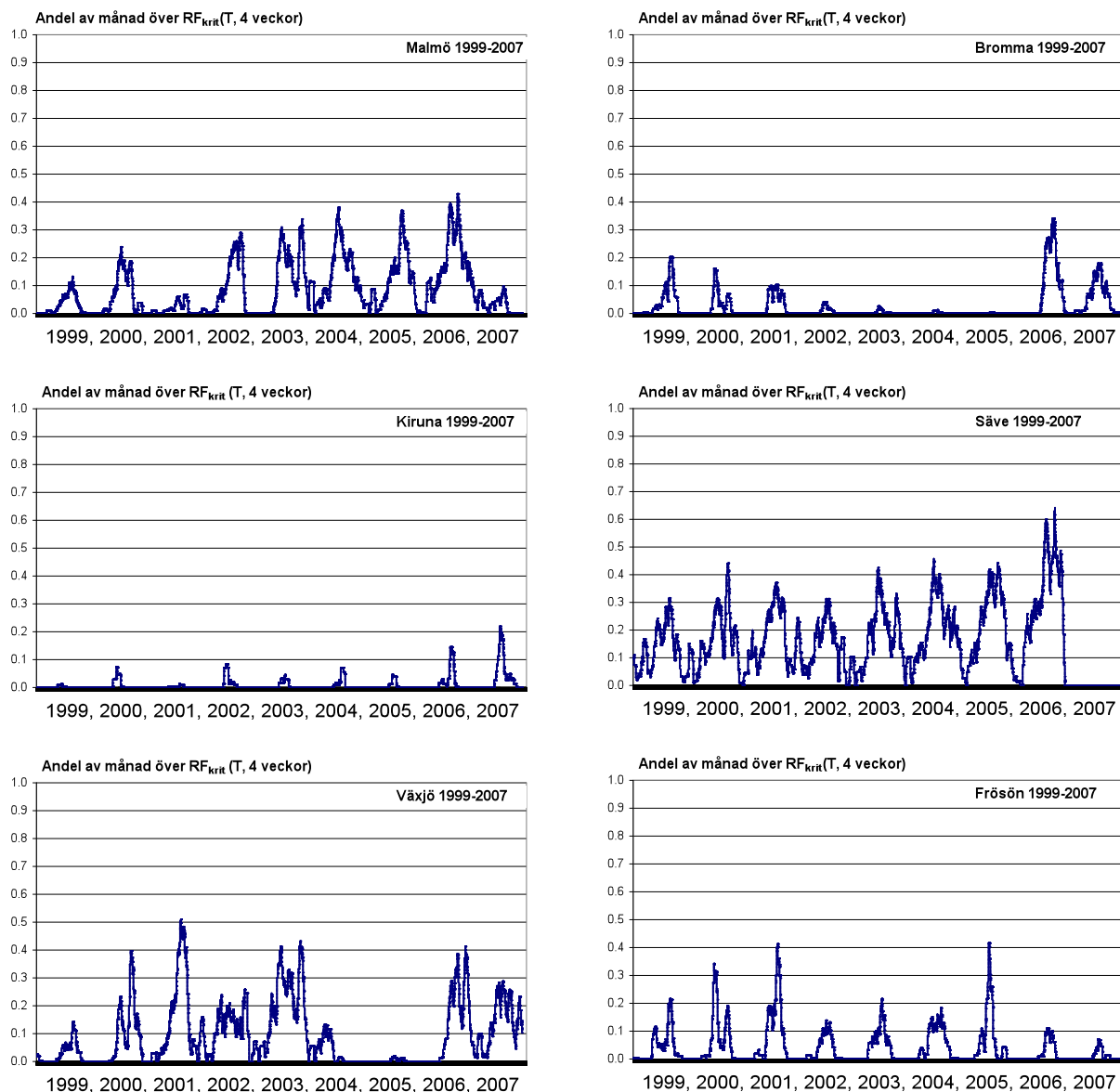
Fig. 8.6 Sammanlagd varaktighet under en månad av RF(T) över den kritiska RF_{krit}(T,t) för varaktigheten en månad, som andel av en månad. Olika orter i Sverige 1999-2007
