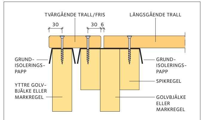
Figur 6 Tvärgående trall, så kallad fris, monteras för att dölja ändträytor på trädäckets kortsidor. Extra stöd genom påsalning av spikreglar innanför den yttre golvbjälken eller markregeln. Trallbrädor ska monteras med 6 mm bred rörelsefog mot fris.
